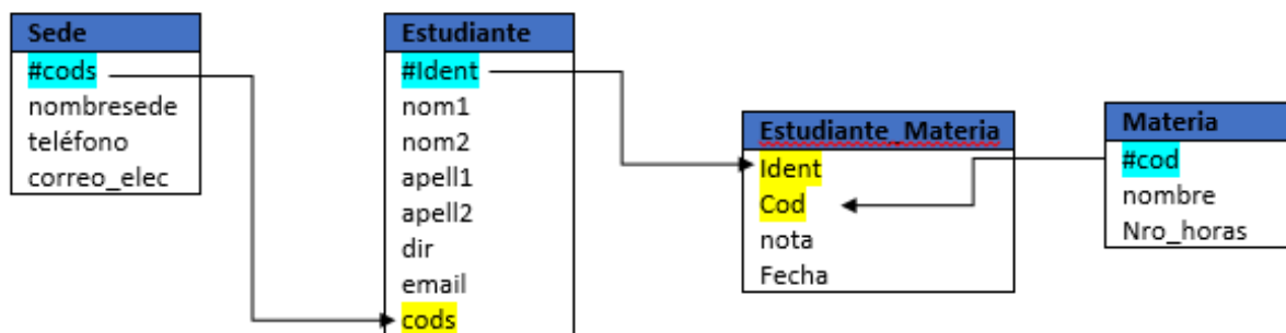
Imagen 18 Modelo Relacional
